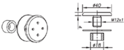
Front cylindrisk, for 20 til 100 mm.
