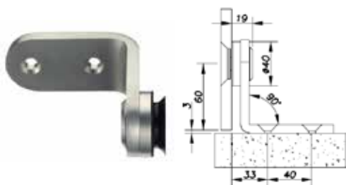
Vinkel 90°
