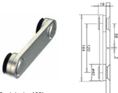
Samle beslag 180°
