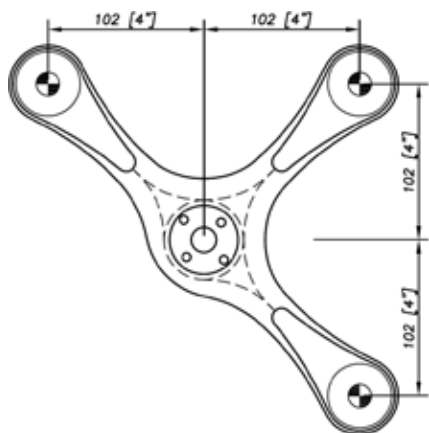
3 armet spider
