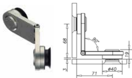
Juster bar vinkel 90 - 180°
