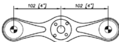
2 armet spider
