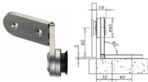
Juster bar vinkel 90 - 180°
