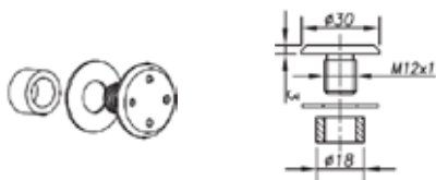
Front cylindrisk, for 20 til 100 mm.
