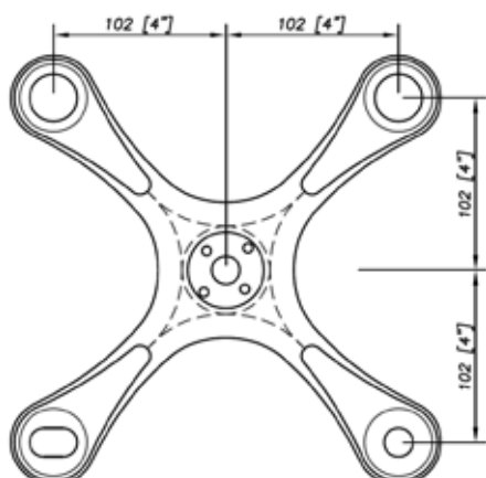
4 armet spider
