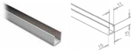
U-profiler 15x15x15 mm.
