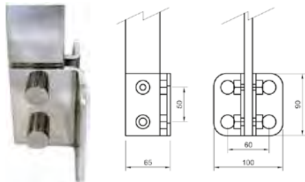
Sidemonteret fod
