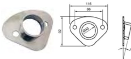
Vægplade til håndliste vinkel
