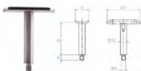
Håndlistestøtte lige
