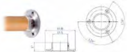
Vægmontageplade
