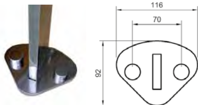
Standart fod
