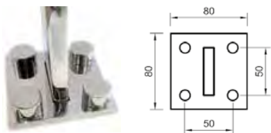
Firkantet fod
