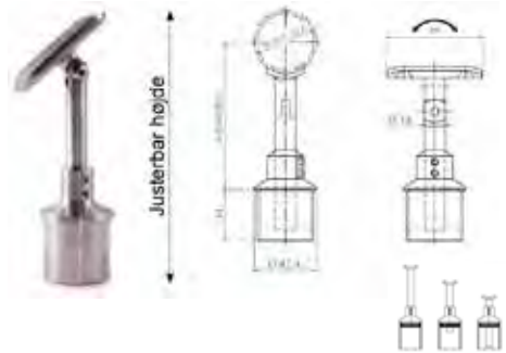
Håndliste holder justerbar højde og vinkel
