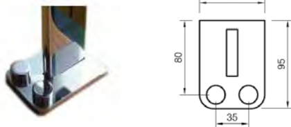
Asymetrisk fod
