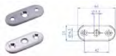
Top flad
