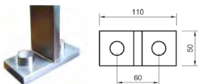
Rektangulær fod
