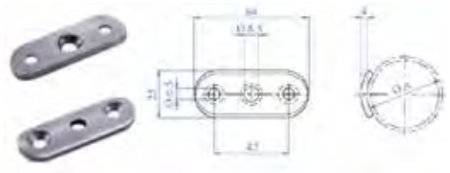
Top lige
