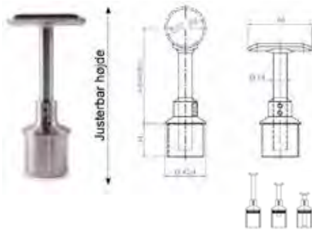
Håndliste holder justerbar højde
