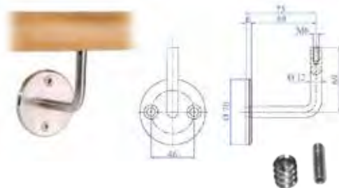
Vægbeslag uden top, monteres i træet.
