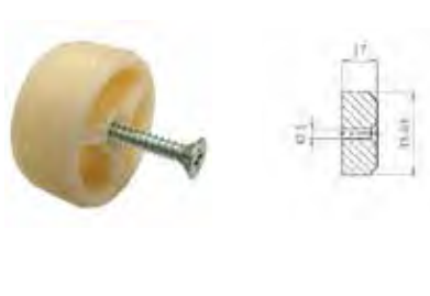
Plastic beslag, til endepapper og samleled.
