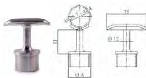
Håndlistestøtte 50 mm.
