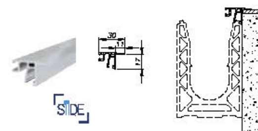
Dækkappe NOT T3 miks tætning mod mur - Én sidet
