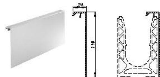
Side dækkappe G12 & G19 - To sidet
