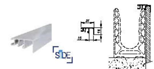
Dækkappe NOT T10 miks tætning - Én sidet
