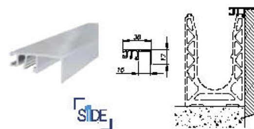
Dækkappe NOT T15 miks tætning - Én sidet
