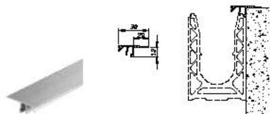
Top dækkappe overgang gulv - To sidet
