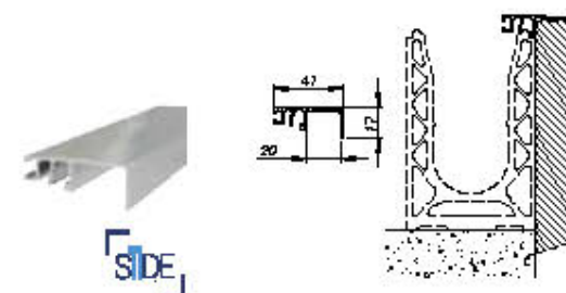
Dækkappe NOT T20 miks tætning - Én sidet
