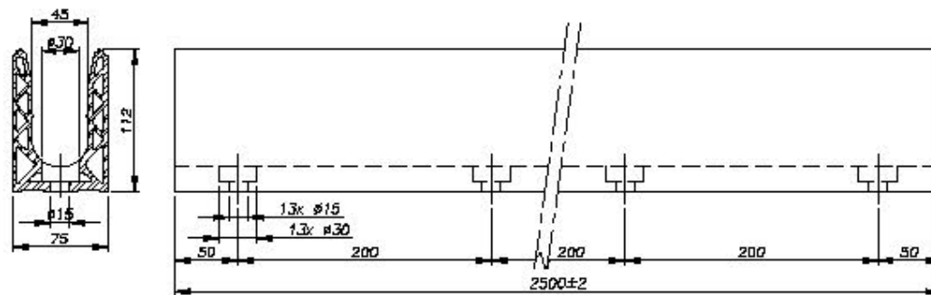
TL1515 ORIGINAL® sidemonteret - profilsnit
