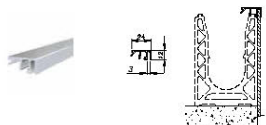
Dækkappe NOT T3 - To sidet
