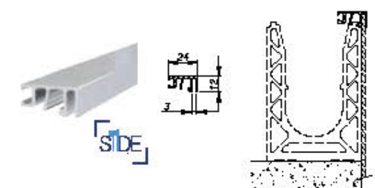
Dækkappe NOT T3 miks tætning - Én sidet
