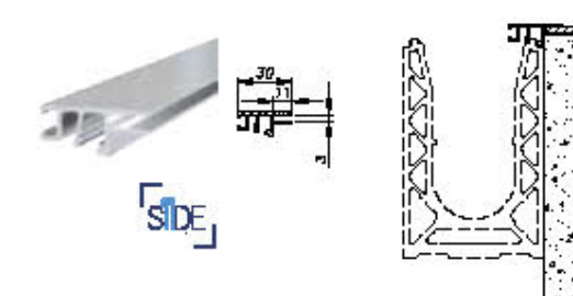
Dækkappe NOT T3 miks tætning - Én sidet
