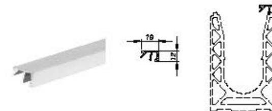
Lille top dækkappe - To sidet
