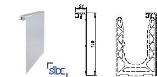
Side dækkappe miks tætning - Én sidet
