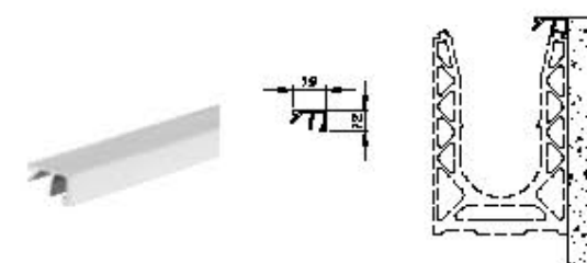
Lille top dækkappe mod mur - To sidet
