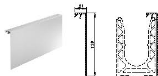
Side dækkappe - To sidet
